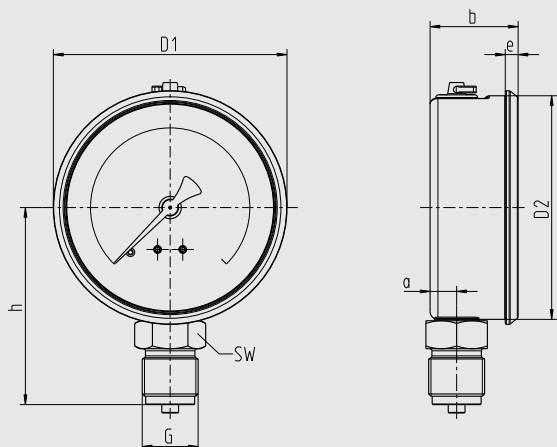
DN 80, attacco al processo inferiore (LM)
