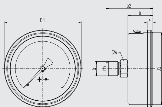
DN 100, attacco al processo posteriore centrale (CBM)
