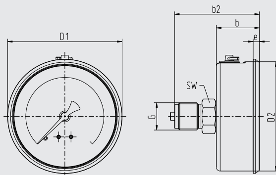
DN 80, attacco al processo posteriore centrale (CBM)
